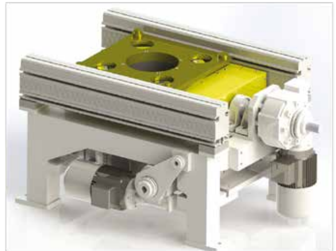
Pallet Lift & Turning unit for motor and gearbox assembly lines Rotosollevatore pallet per linee di montaggio motore e cambio
